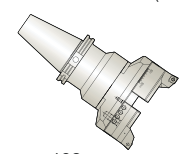
DIN 69871-SK (TWIN TBH)
